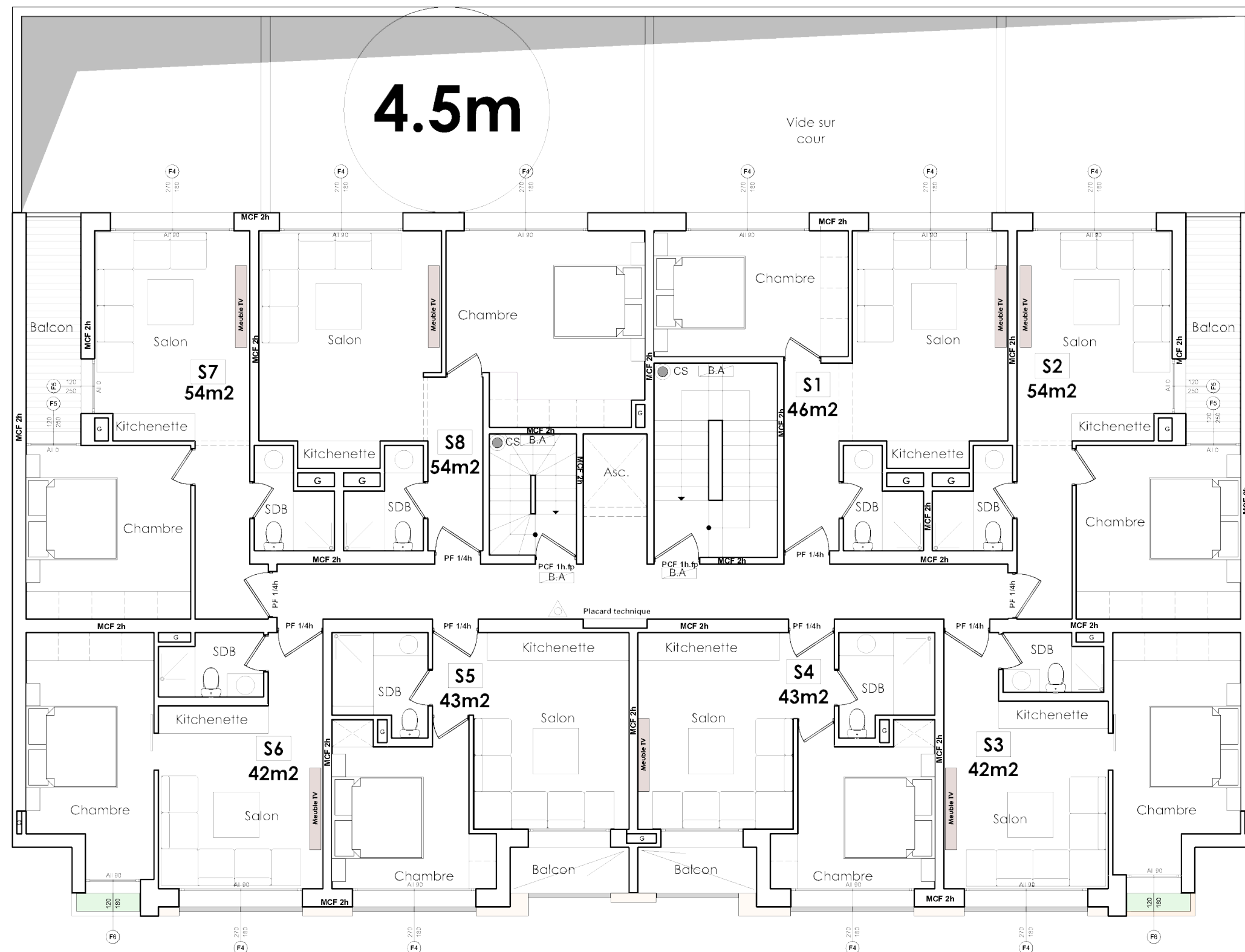
ETAGE COURANT (1/2/3) SUPERFICIE COUVERTE : 410m2
