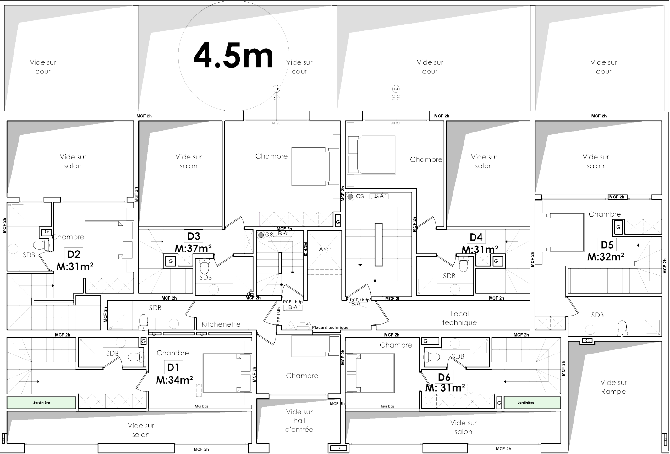
MEZZANINE SUPERFICIE COUVERTE : 250m2
