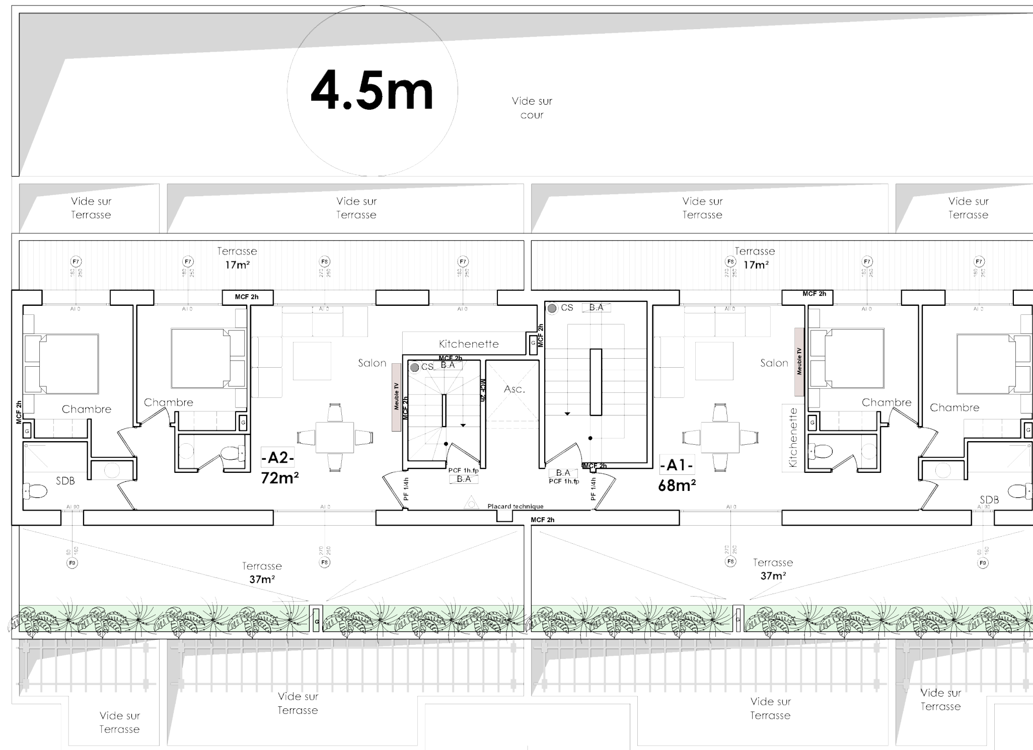
5e ETAGE SUPERFICIE COUVERTE : 170m²
